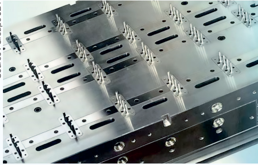
Moule multi-empreintes conçu et fabriqué par Groupe JBT
